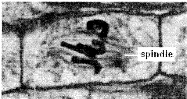
Metaphase
